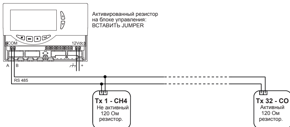
Рис. 6: Пример соединения : Блок контроля - сенсор
